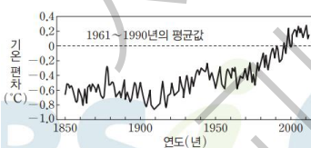
지구의 기온 변화
