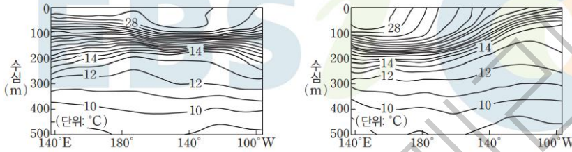
엘니뇨(왼쪽)와 라니냐(오른쪽) 발생 시 열대 태평양의 해수 온도의 연직 분포
