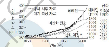
온실 기체의 농도 변화
